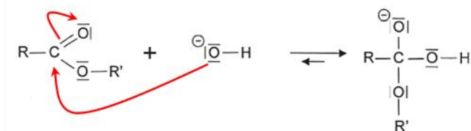
Figure 2. Mécanisme de réaction
