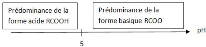
Figure 3. Diagramme de prédominance
